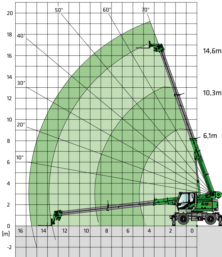
Lifting fork 6,1-14,6
